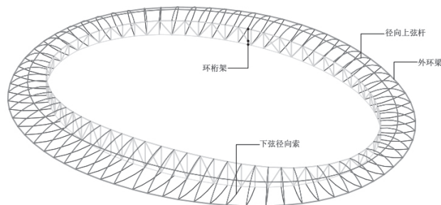
▲非对称大跨度索承空间结构体系轴测图
